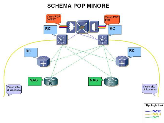
Figura 3. Schema architetturale di un PoP minore
