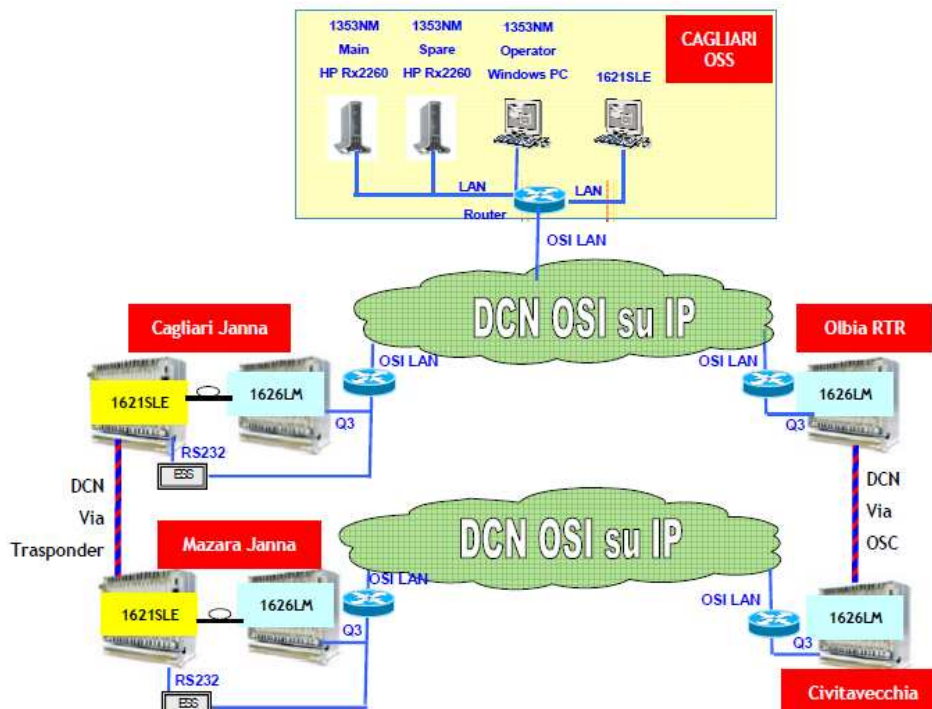
Figura 6. Architettura generale dei sistemi di illuminazione delle tratte sottomarine
