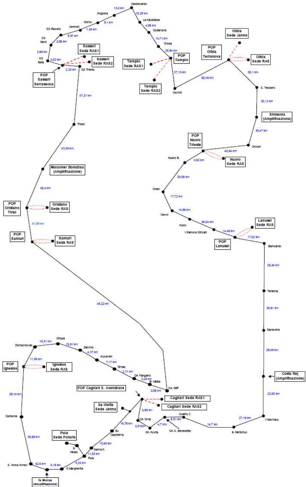
Figura 1. Sviluppo dell'infrastruttura su fibra ottica della RTR
