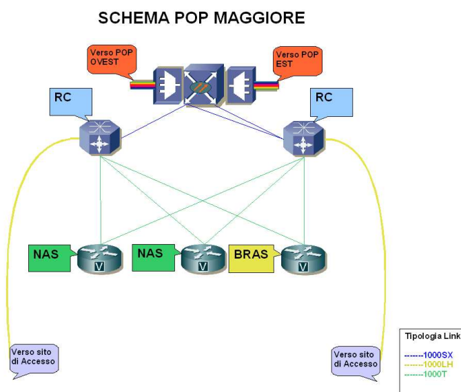
Figura 2. Schema strutturale di un PoP maggiore
