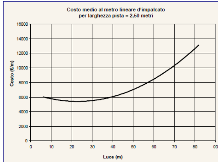
Figura 0.1 – Costo d'impalcato
